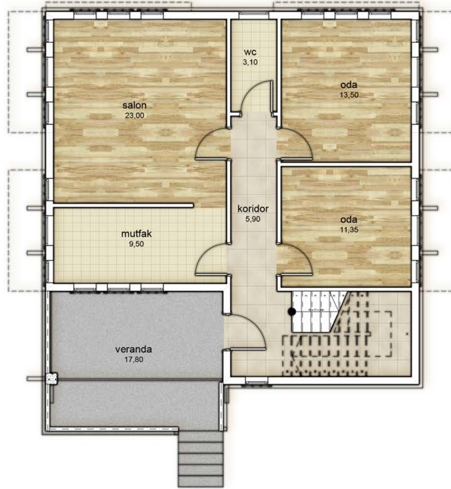
Tip 15 : Zemin Kat Planı
