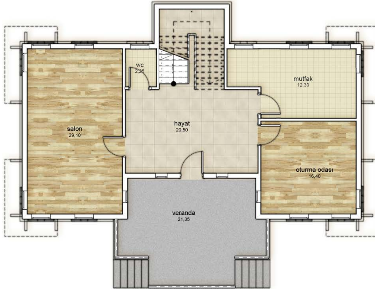
Tip 17 : Zemin Kat Planı
