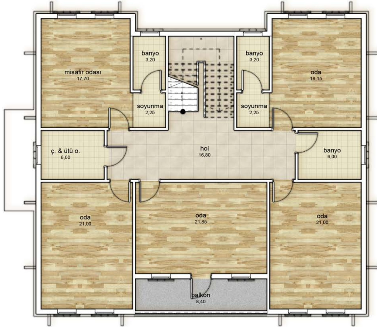
Tip 22 : Birinci Kat Planı
