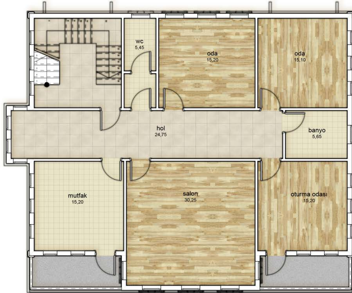
Tip 11 : Birinci Kat Planı
