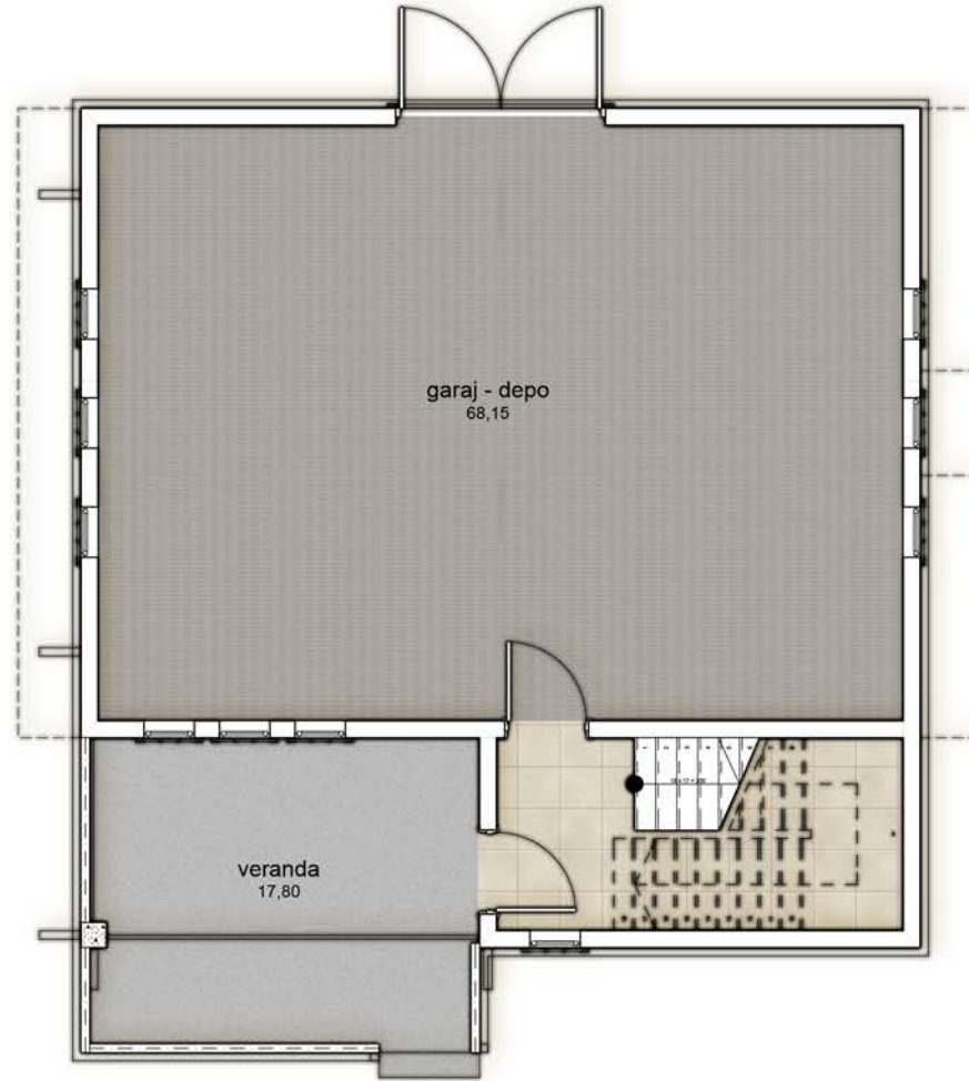
Tip 09 : Zemin Kat Planı
