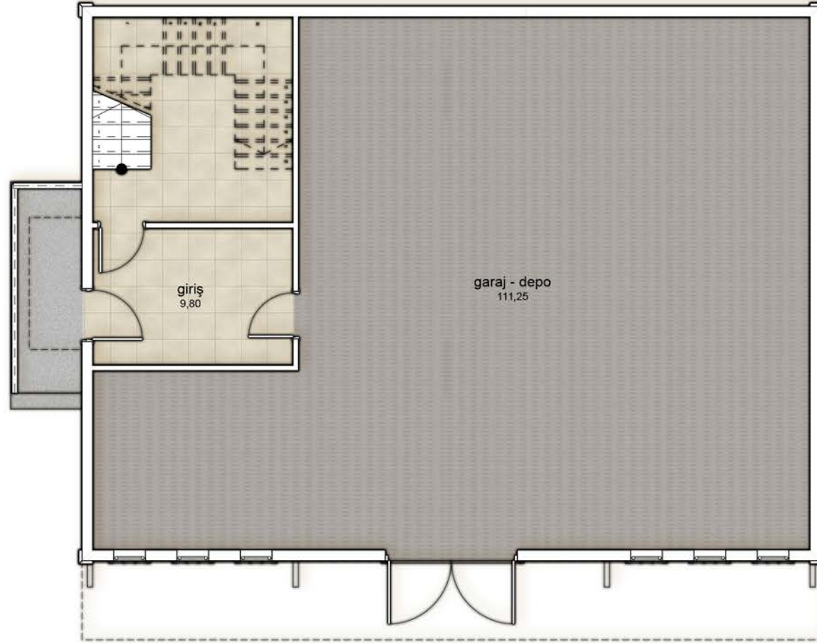
Tip 11 : Zemin Kat Planı
