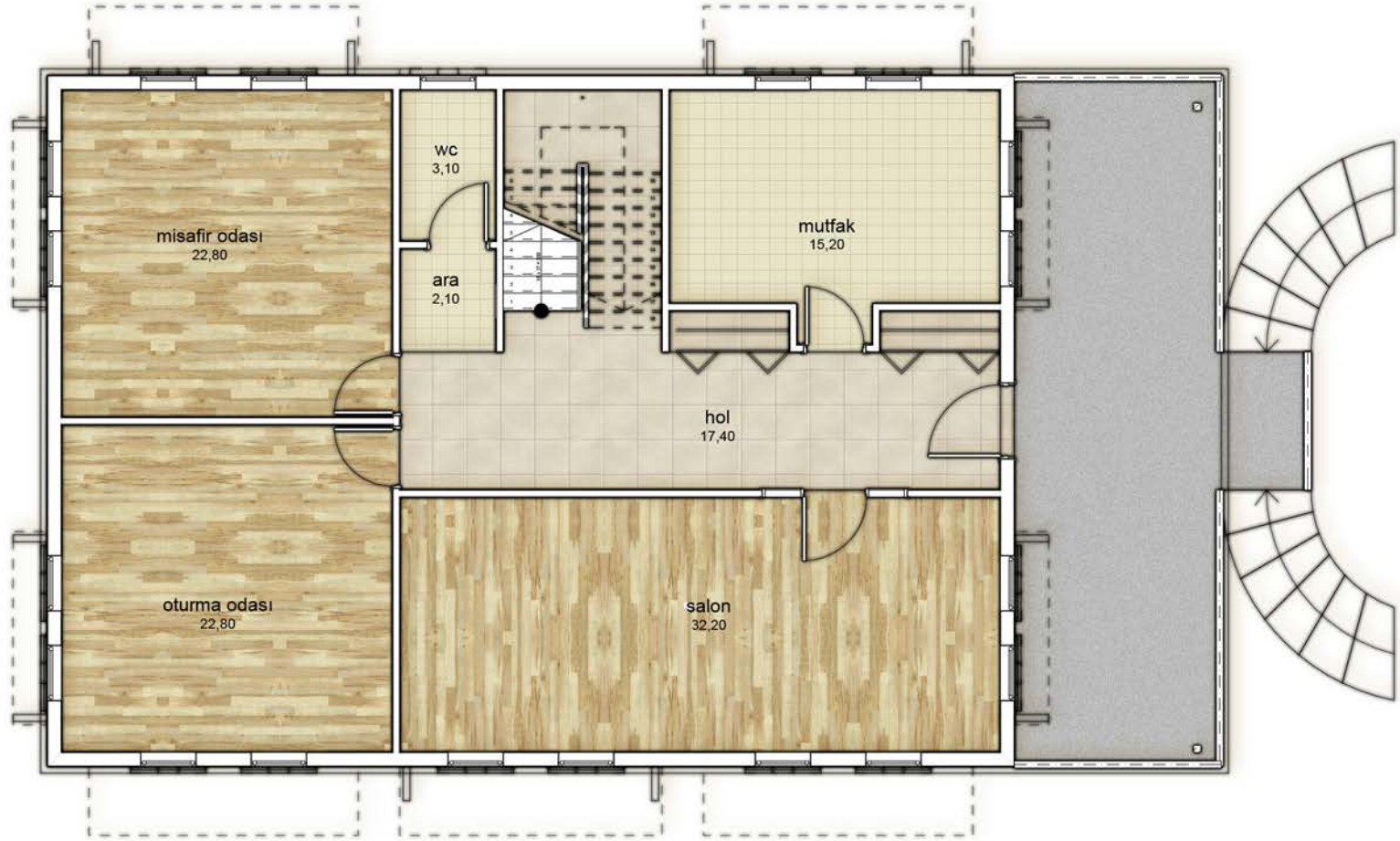
Tip 20 : Zemin Kat Planı
