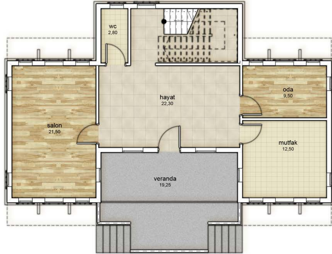
Tip 16 : Zemin Kat Planı
